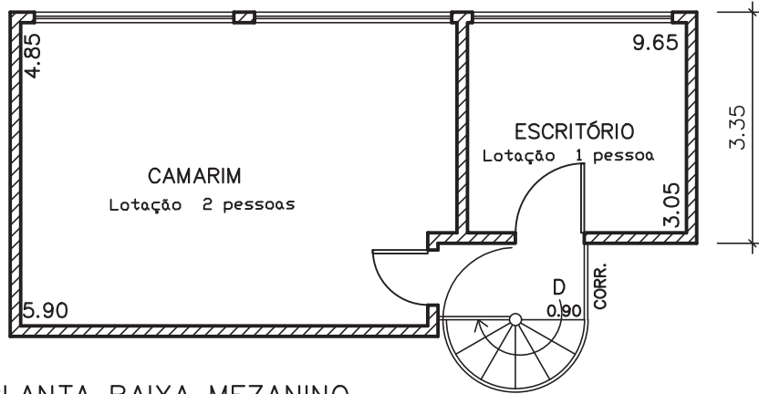
PLANTA BAIXA MEZANINO ESC: 1/100
